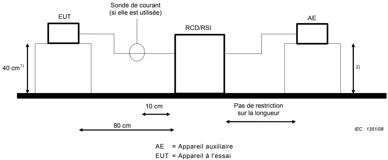
Figure C.1 – Utilisation du RCD décrit dans la CEI 61000-4-6 en tant que RCD/RSI
