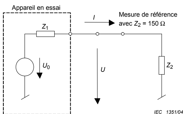
Figure F.1 – Circuit de base pour la considération des limites avec une impédance TCM définie de 150 Ω
