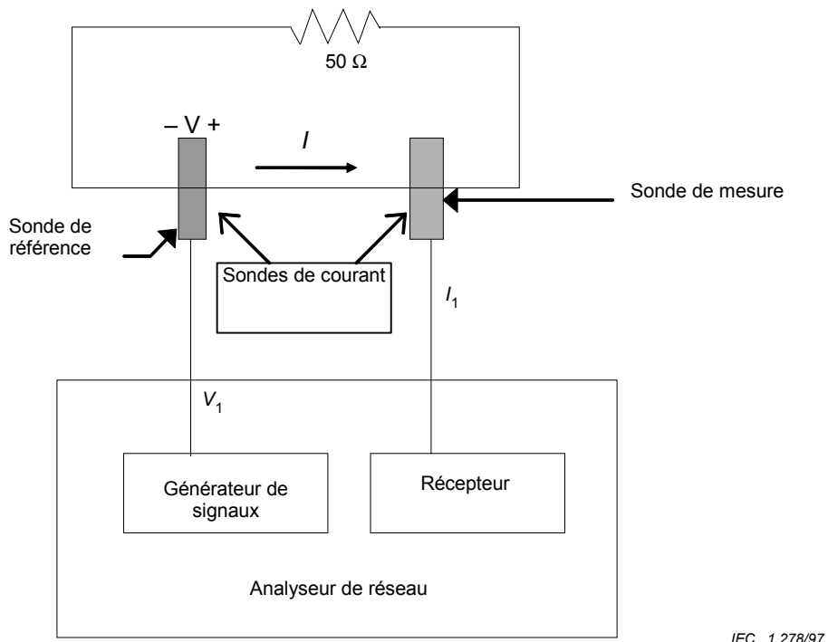
Figure C.4 – Dispositif d'étalonnage
