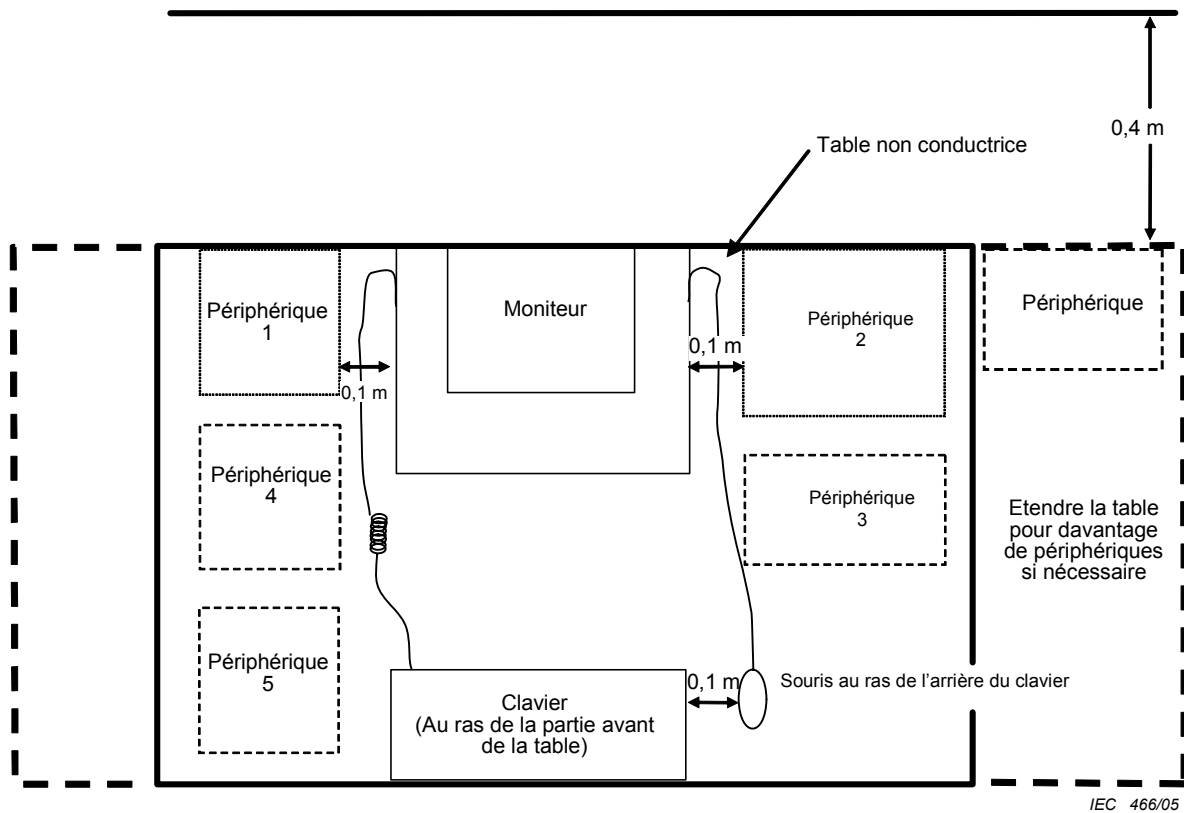
Plan de masse de référence vertical (émissions conduites uniquement – variante 1)
